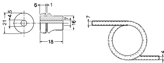
Fig. 5 Kit para montaje en conducto, nº de pieza GMT008N600R
